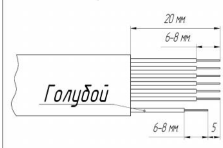
Схема обрезки кабеля
